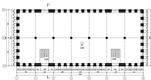
План здания на уровне +0,000 м
