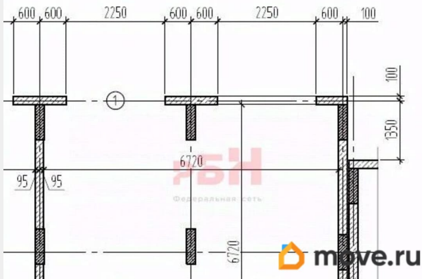
Кладочный план
